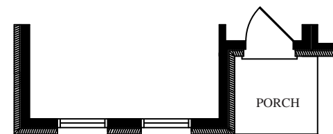
ELEV. B
